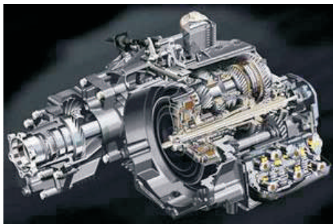
Fig: Gear Box
